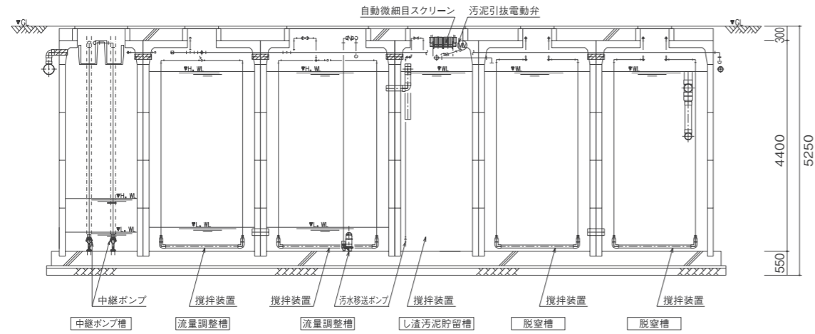
A-A断面図
