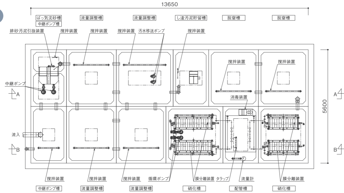
平面図
