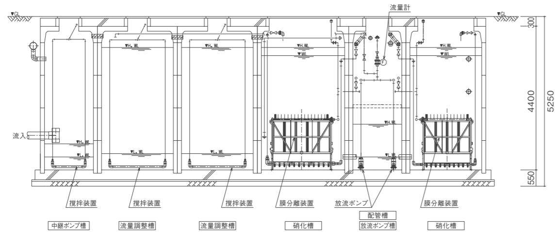
B-B断面図
