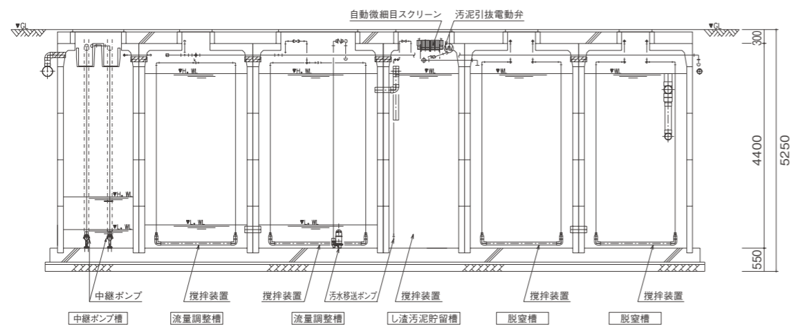
A-A断面図
