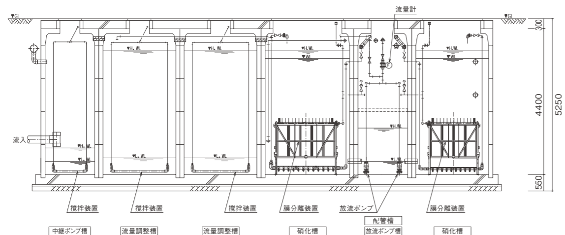
B-B断面図
